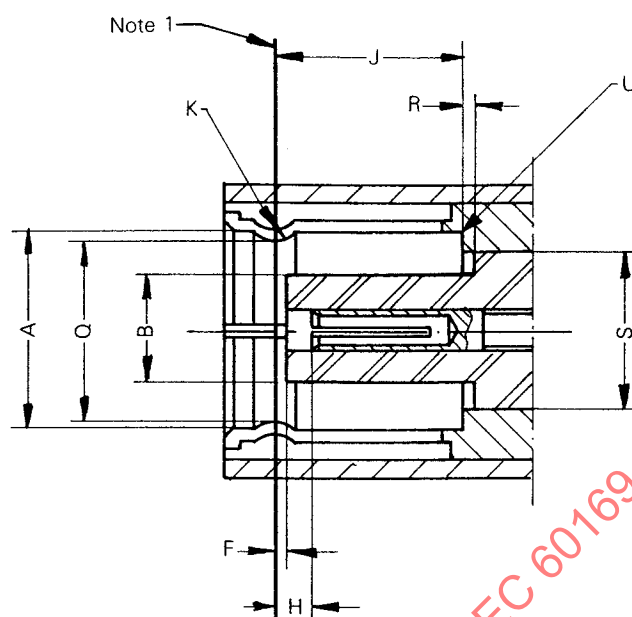
FIG. 6A. — Dimensions du connecteur (voir tableau). Dimensions of connector (see table).
