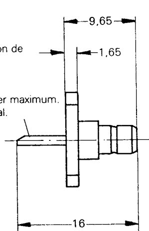
FIG. 11. — Embase à platine (fixation sur panneau par quatre trous avec cosse à souder) avec contact mâle.
