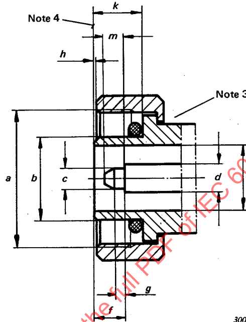
FIG. 1. — Connecteur avec contact central mâle (pour les dimensions, voir le tableau) Connector with pin centre contact (for dimensions see table)
