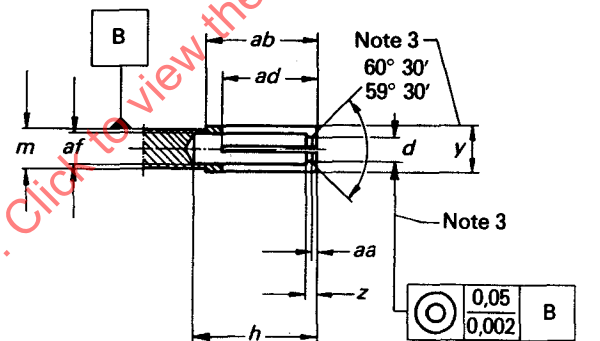
FIG. 6B. — Dimensions du contact central femelle (voir le tableau). Dimensions of centre contact (see table).
