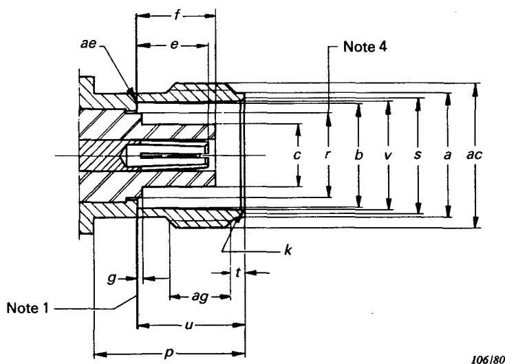
FIG. 2A. — Connecteur avec contact central femelle (pour les dimensions, voir le tableau). Connector with socket-centre contact (for dimensions, see table).
