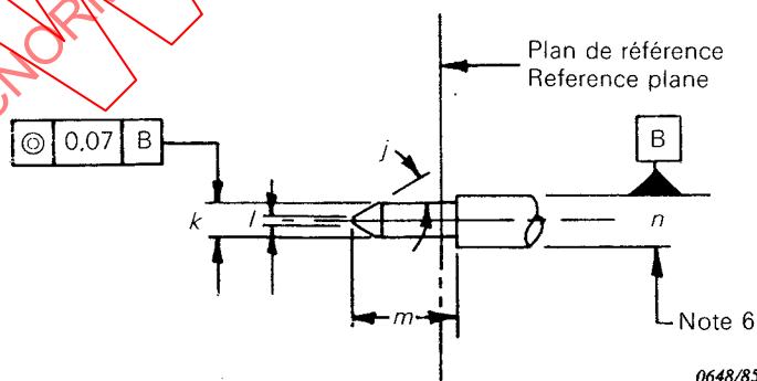
FIG. 7. — Détails du contact central mâle. Details of female centre contact.
