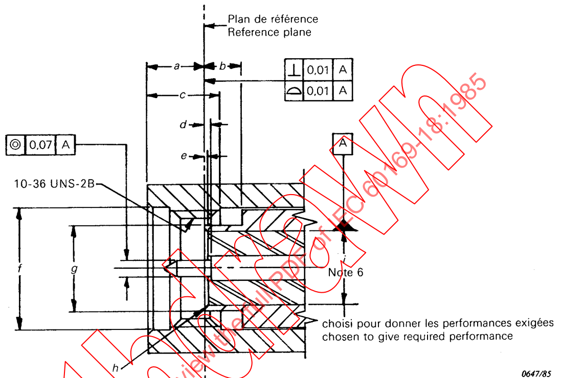
FIG. 6. — Fiche (contact mâle). Plug (male contact).
