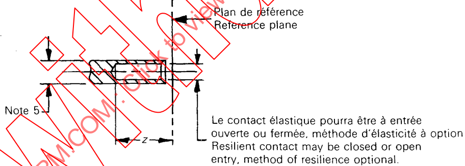
FIG. 4. — Détails du contact central femelle élastique. Details of female centre resilient contact.
