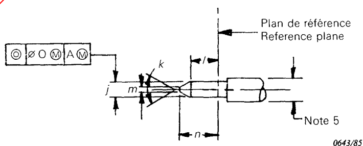
FIG. 2. — Détails du contact central mâle. Details of male centre contact.
