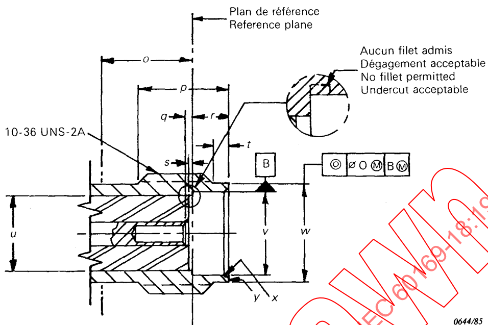
FIG. 3 — Prise (contact femelle). Socket (female contact).
