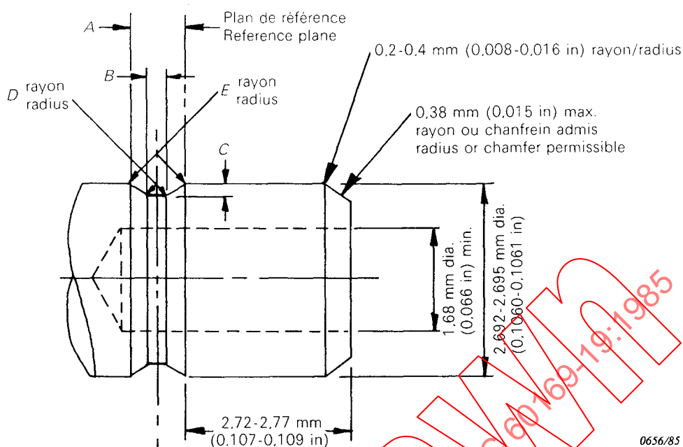
FIG. 6. — Calibre A et B pour le calibrage du contact extérieur et la mesure de la force de rétention (pour les dimensions voir tableau). Outer contact sizing and retention force gauges A and B (for dimensions see table).
