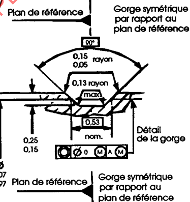
Figure 2c - Détails de la gorge d'accouplement
