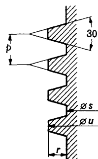
FIG. 4. — Détail du filetage. Detail of screw thread.
