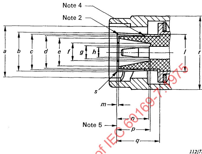
FIG. 7. — Dimensions du connecteur (voir le tableau). Dimensions of connector (see table).
