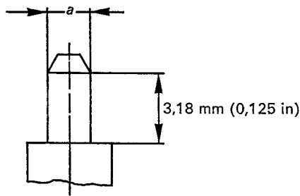
FIG. 5. — Calibre (broches) pour contact central du connecteur femelle. Gauge (pins) for centre contact of socket connector.
