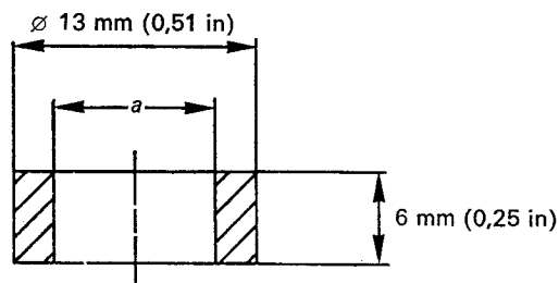
FIG. 4. — Calibre (anneau) pour contact extérieur du connecteur mâle. Gauge ring for outer contact of pin connector.
