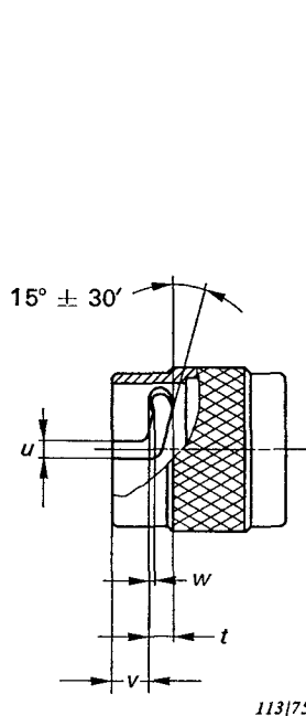
FIG. 8. — Dimensions du verrouillage à baïonnette (voir le tableau). Dimensions of bayonet lock (see table).
