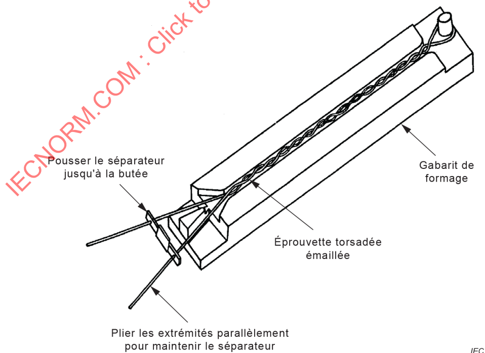
Figure 4 – Éprouvette disposée dans le gabarit de formage
