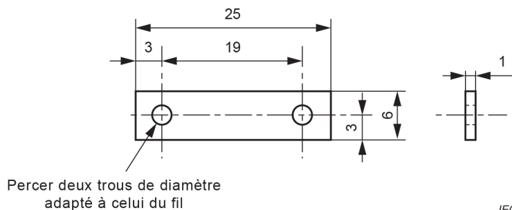
Figure 2 –Séparateur
