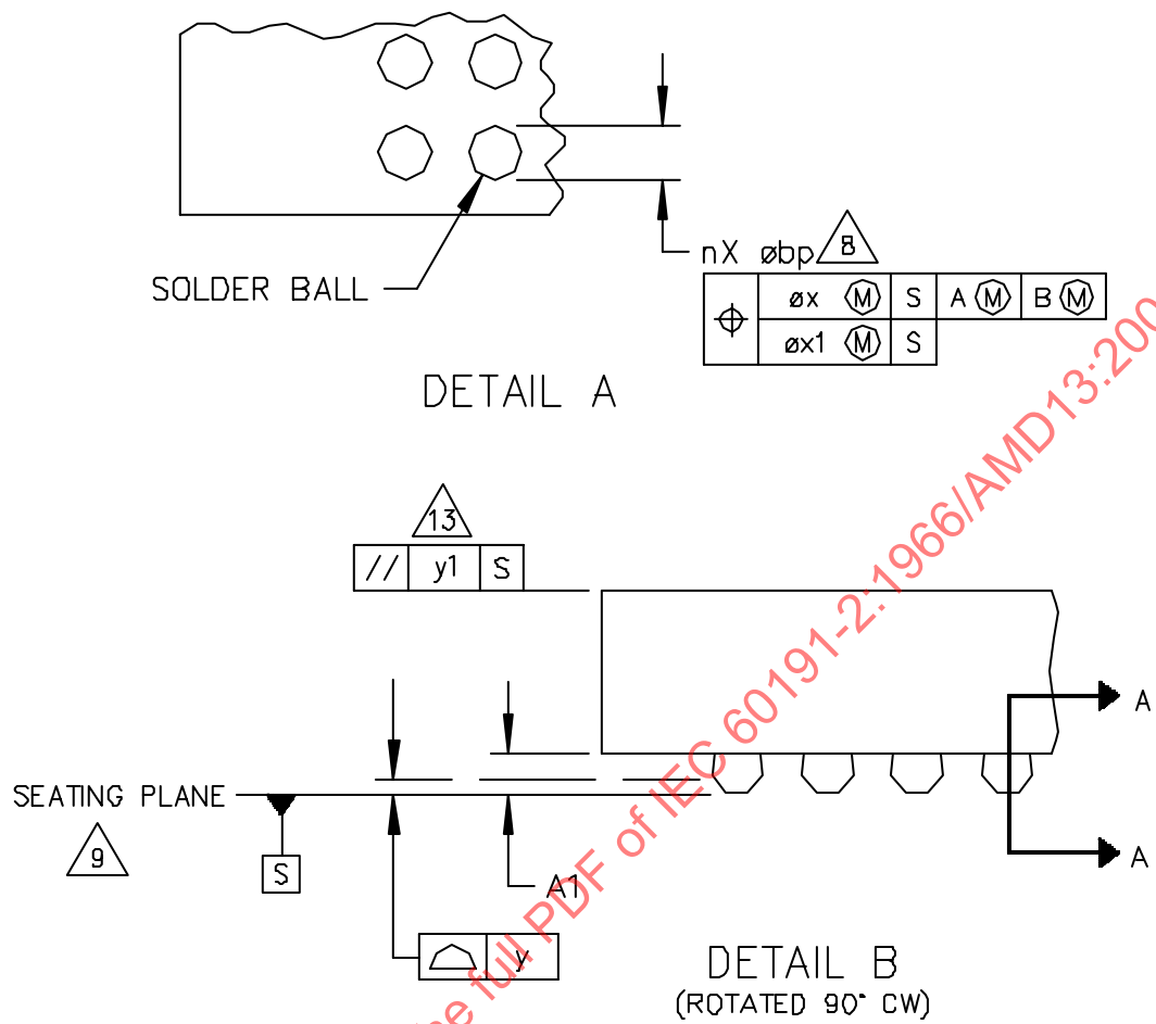
SECTION A-A
