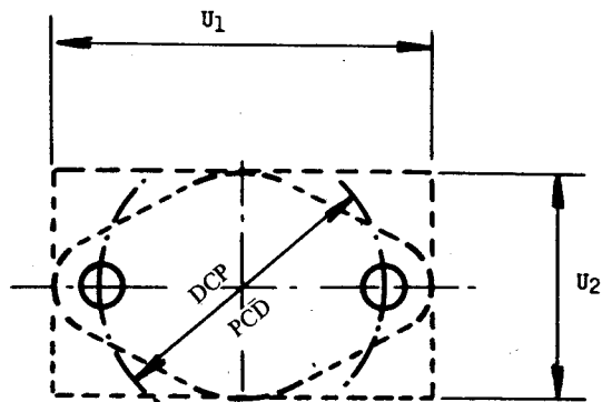
Fig. 1. — Encombrements d'embases plates en forme de losange ou de rectangle. Outlines of lozenge or rectangular shaped flat bases.
