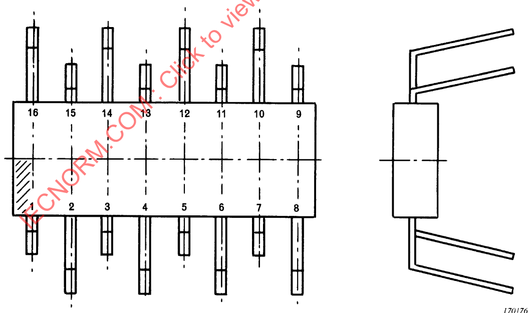
Figure 3 – Exemple montrant comment numéroté les sorties d'un boîtier «QUIL»
