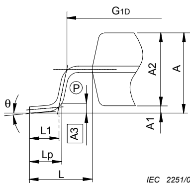
Figure 1d – Vue de côté du conducteur
