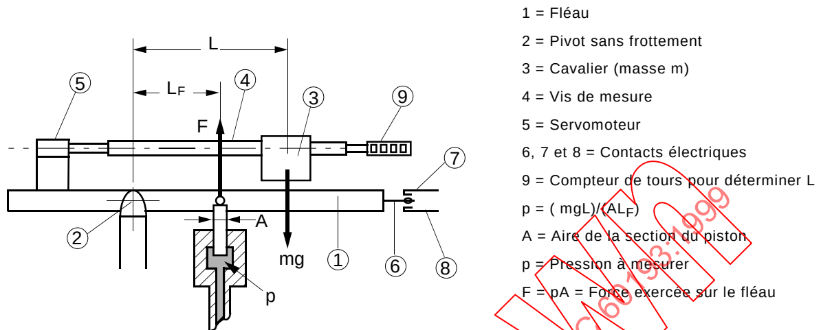
Figure 35 – Balance de pression (exemple de montage expérimental)
