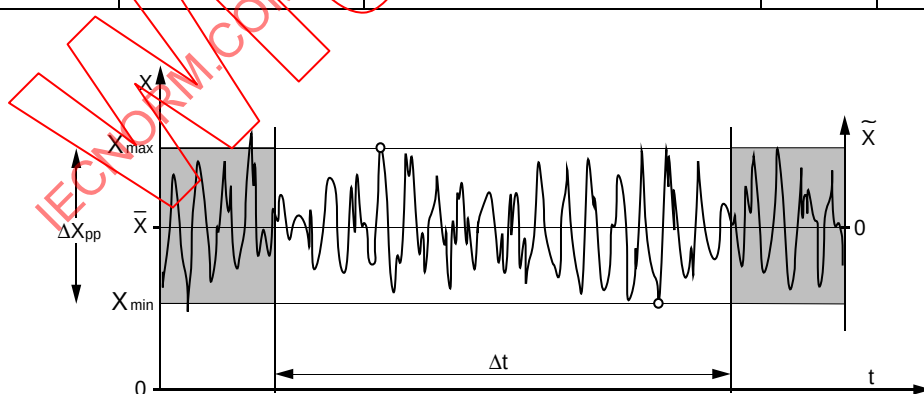
Figure 7 – Illustration de quelques définitions relatives aux grandeurs fluctuantes
