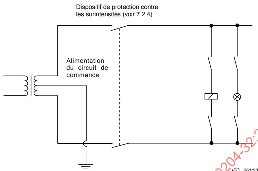
Figure 6 – Protection contre des manœuvres impropres dues à des défauts à la terre – Méthode b)
