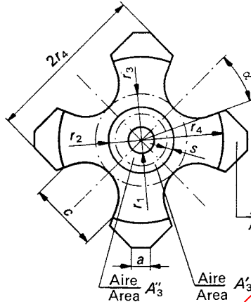
Noyau-X à jambes arrondies X-core with rounded legs
