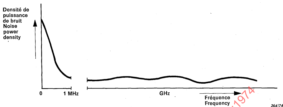
FIG. 18. — Répartition du bruit de fond en fonction de la fréquence. Frequency distribution of background noise.
