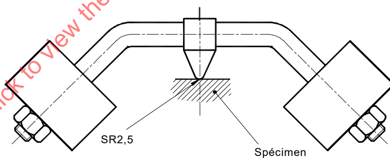
Figure 9 – Appareil pour la résistance à la compression
