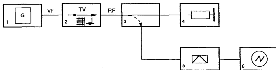
Figure 2a – Montage de mesure pour déterminer la stabilité et les niveaux, des signaux caractéristiques et de l'écrêteur de blanc Measuring arrangement for setting white clipper and characteristic levels and for stability measurement
