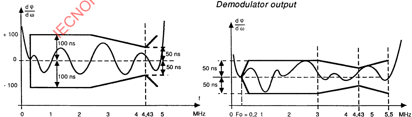
Figure 3h – Exemples de graticules pour la mesure du temps de propagation de groupe des standards L et G Examples of group-delay graticule for systems L and G
