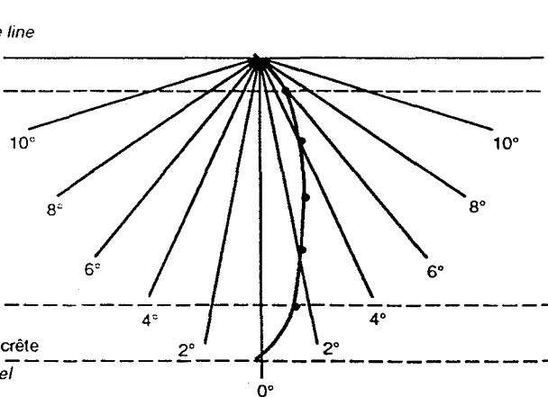
Figure 4g – Montage pour la mesure de la modulation de la phase incidente Measuring arrangement for incidental phase modulation
