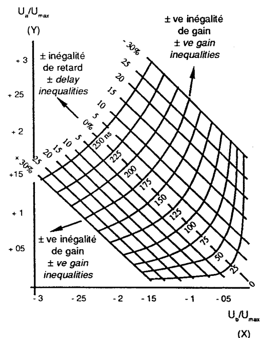
Figure 5o – Inégalité de retard et de gain chrominance/luminance Chrominance-luminance gain and delay inequality
