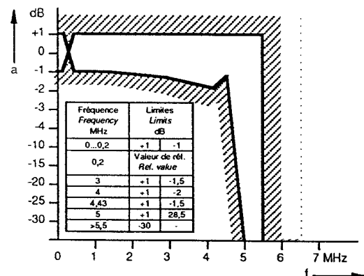
Figure 3e – Exemple de caractéristiques amplitude/vidéofréquence avec tolérances pour le standard G Example of amplitude/video-frequency characteristics with tolerance for system G
