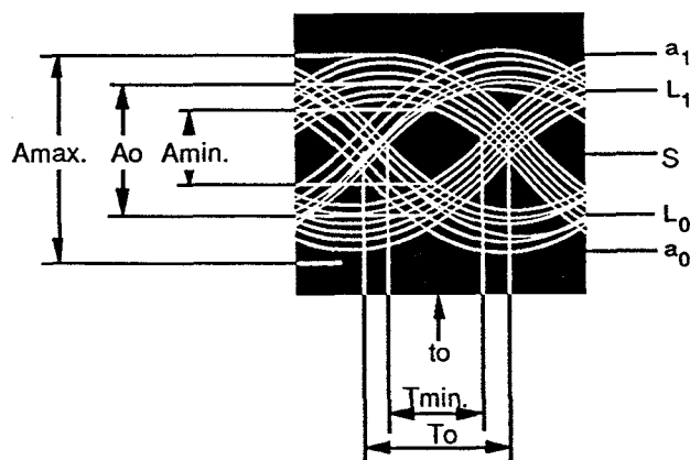
Figure 7a – Hauteur de l'oeil et largeur de l'oeil Eye-height and eye-width
