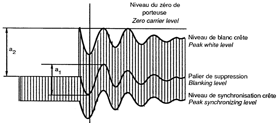
Figure 5n – Suroscillation due à la variation noir-blanc visualisée à basse fréquence Displayed black to white signal change shows ringing when employing low frequency sweep
