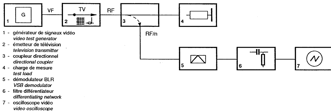
Figure 4a – Montage pour la mesure de non-linéarité de la luminance Measuring arrangement for luminance non-linearity
