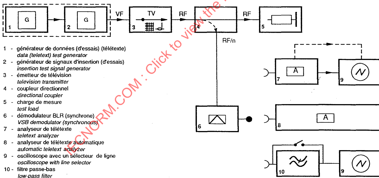
Figure 7b – Montage pour la mesure de la hauteur et de la largeur de l'oeil Measuring for eye-height and eye-width
