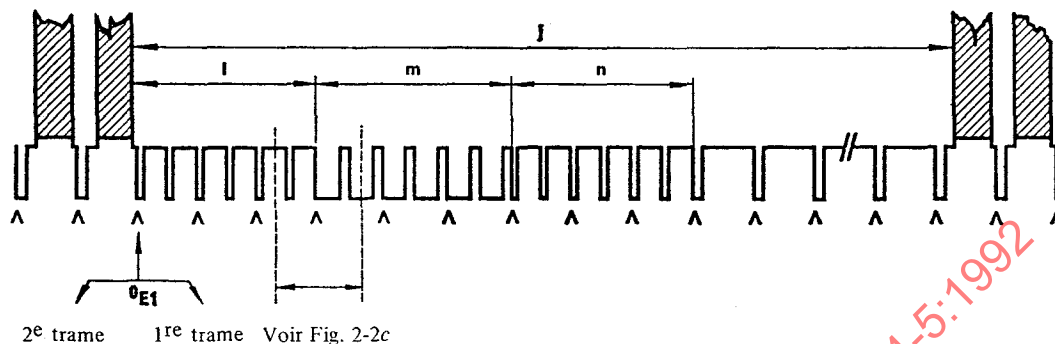
FIGURE 2-2a – Signal au début de chaque 1 re trame
