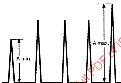
Figure 4b – Sortie démodulée après filtre différentiateur Differentiated demodulator output
