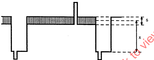
Figure 3b – Sortie démodulée Demodulator output
