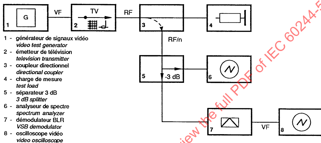
Figure 6b – Montage pour la mesure des produits d'intermodulation et des composantes monofréquence parasites Measuring arrangement for intermodulation products and spurious single frequency components
