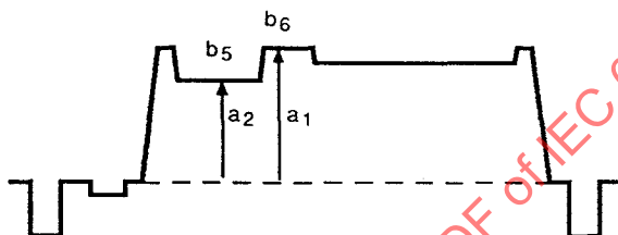
Figure 4f – Sortie démodulée filtrée Filtered demodulator output
