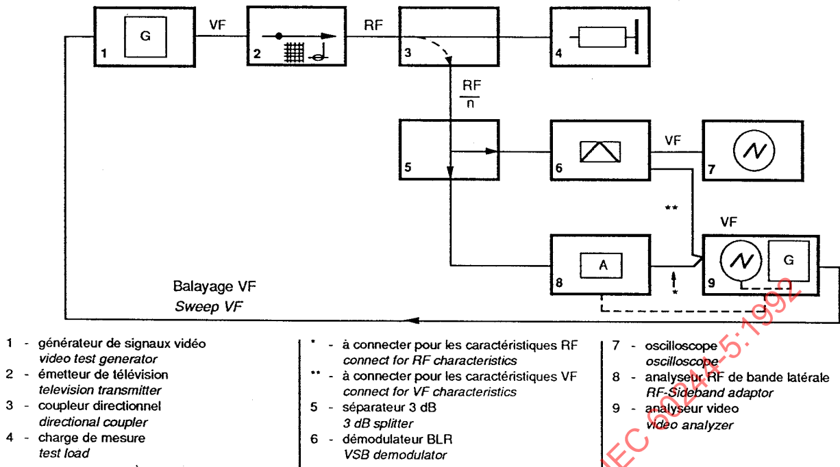
Figure 3a – Montage pour la mesure des caractéristiques amplitude/fréquence Measuring arrangement for amplitude/frequency characteristics
