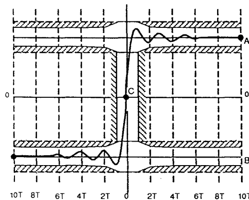
Figure 5g – Echelon de temps de montée T Displayed T step signal
