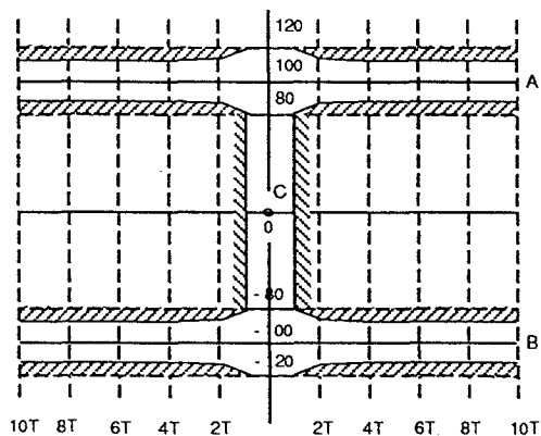
Figure 5f – Graticule pour un échelon de temps de montée T Graticule for T step signal
