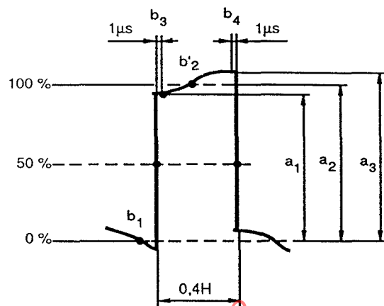
Figure 5i – Signal de barre de luminance de durée ligne Displayed line-time bar signal
