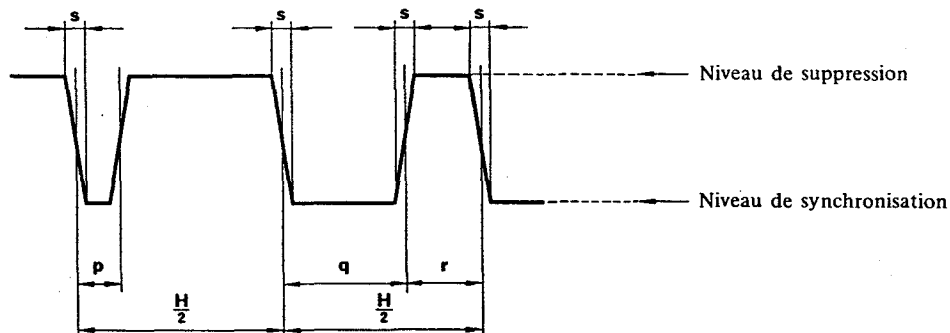
FIGURE 2-2c – Détail des impulsions d'égalisation et de synchronisation
