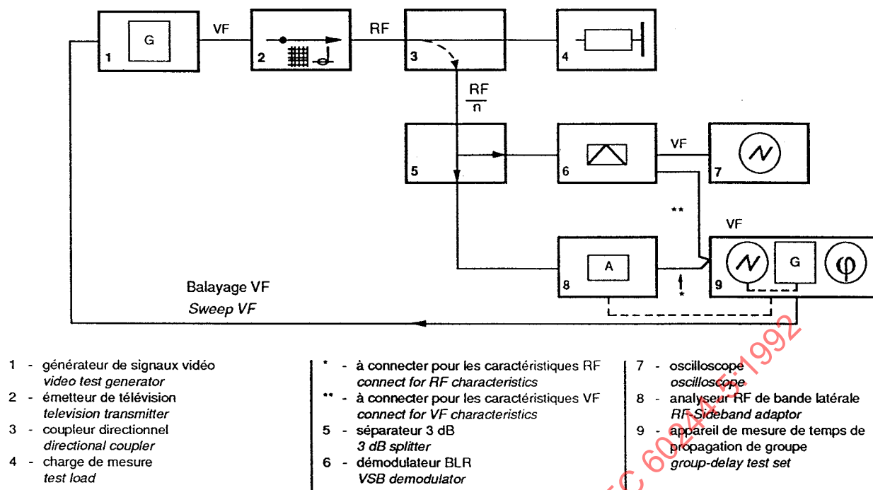
Figure 3f – Montage pour la mesure des caractéristiques temps de propagation de groupe/fréquence Measuring arrangement for group-delay/frequency characteristics
