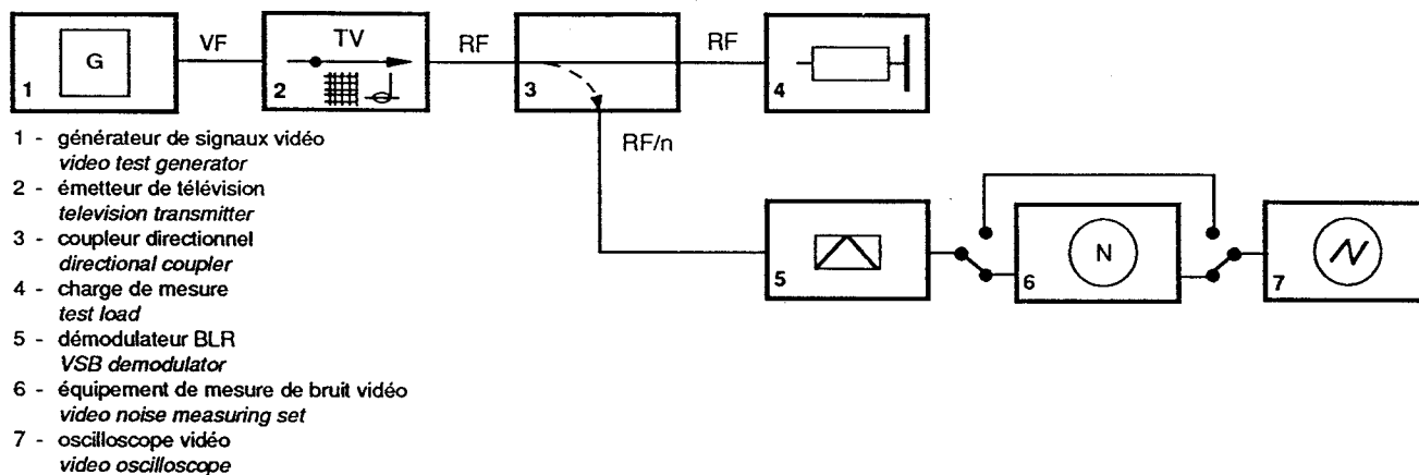
Figure 6a – Montage pour la mesure du rapport signal à bruit Measuring arrangement for signal-to-noise ratio
