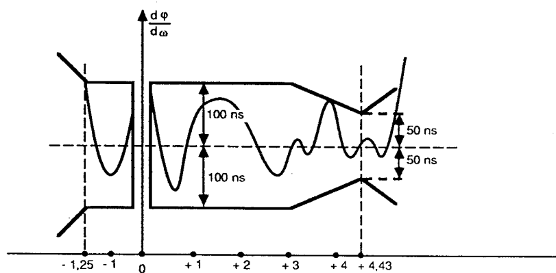
Figure 3i – Exemple de graticule pour la mesure du temps de propagation de groupe du standard G en RF Example of a graticule for RF group-delay characteristics for system G
