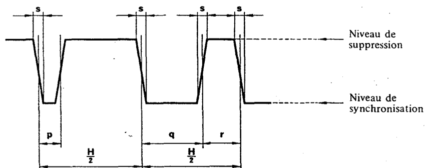
FIGURE 2-1c – Détail des impulsions d'égalisation et de synchronisation
