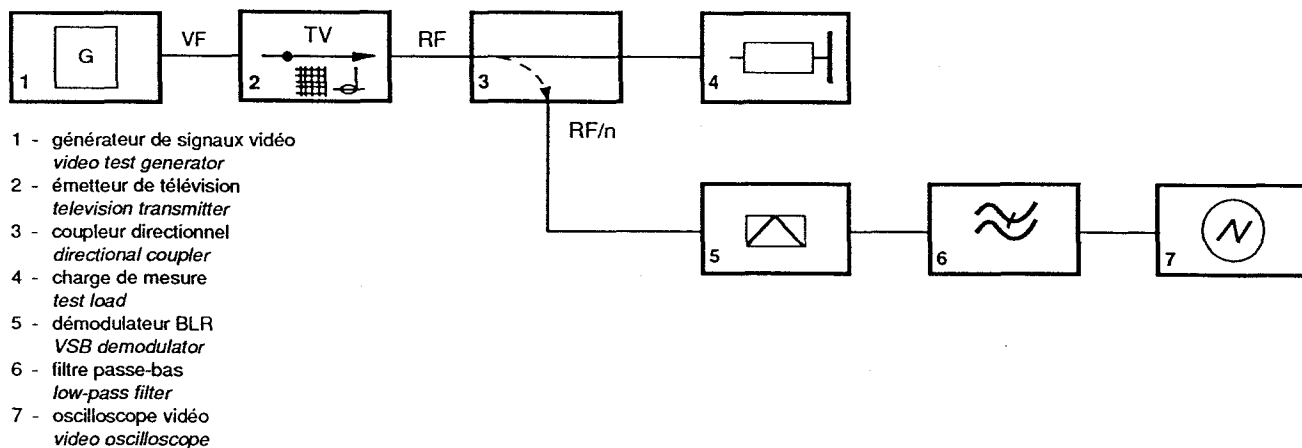
Figure 4e – Montage pour la mesure de l'intermodulation ou de la diaphonie chrominance/luminance Measuring arrangement for chrominance/luminance intermodulation or crosstalk
