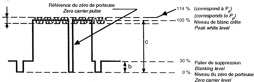
Figures 1b et/and 1c – Signaux en sortie démodulée Demodulator output signals
