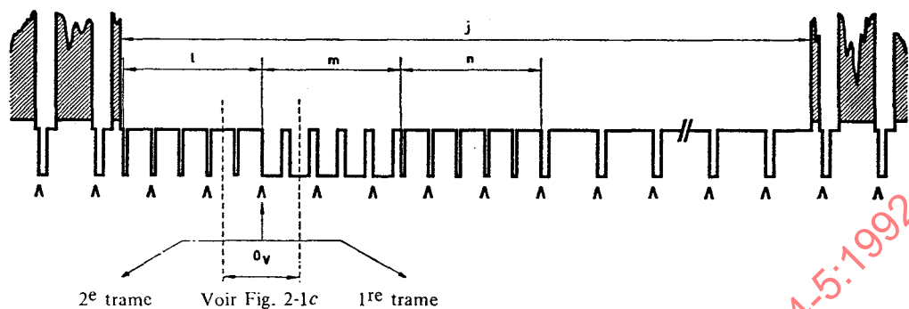
FIGURE 2-1a – Signal au début de chaque 1 re trame
