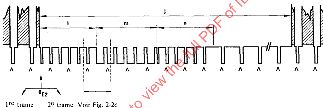
FIGURE 2-2b – Signal au début de chaque 2 e trame
