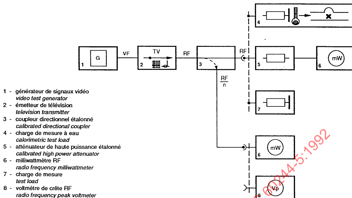
Figure 1a – Montage pour la mesure de la puissance de sortie Measurement arrangement for output power
