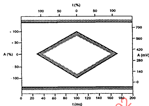
Figure 7c – Mesure en sortie d'émetteur: démodulateur avec réjecteur son (exemple de graticule limite pour le diagramme de l'oeil en détection synchrone) Transmitter output: demodulator with sound trap switched on (example of eye height and eye width graticule with synchronous detection)
