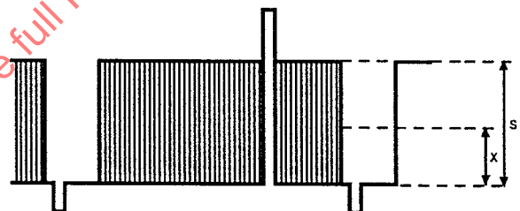
Figure 3c – Sortie démodulée Demodulator output
