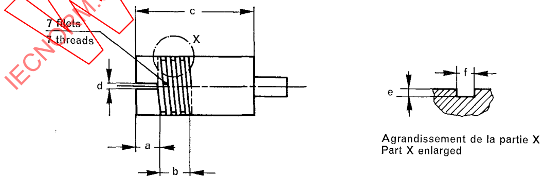
FIG. 2. — Construction et détails du mandrin (voir le tableau IA). Construction and details of the mandrel (see table IA).
