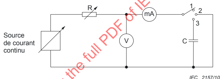
Figure 42 – Dispositif d'essai pour conditionnement en courant continu
