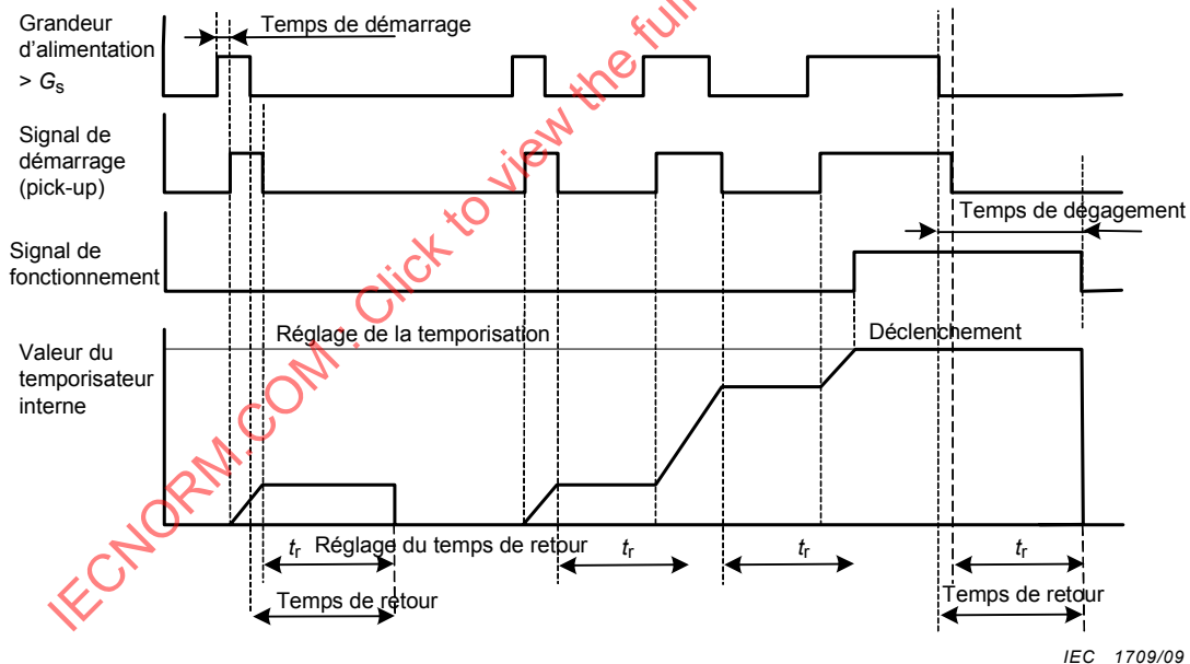
Figure 5 – Caractéristique de retour à temps indépendant
