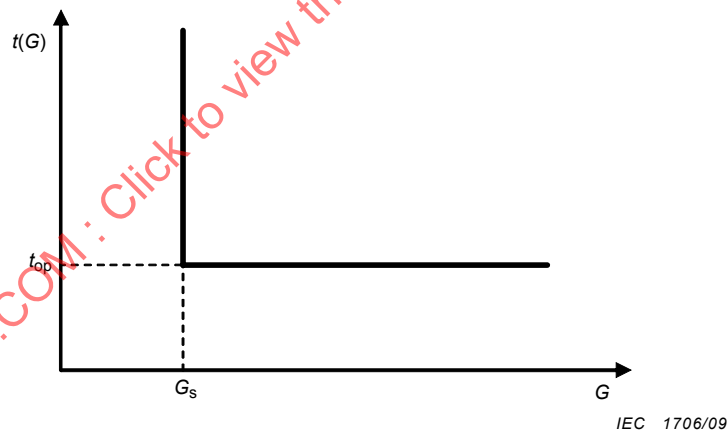
Figure 2 – Caractéristique à temps indépendant à maximum de courant
