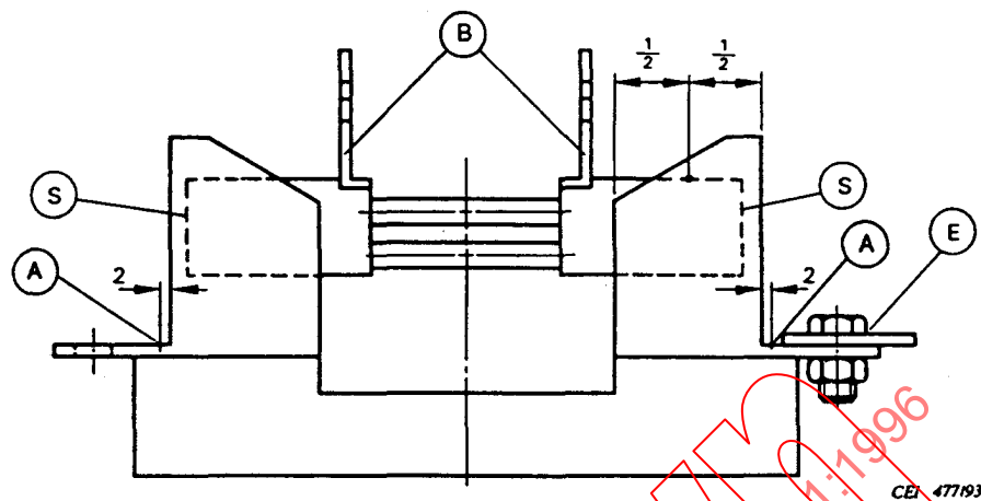
Figure 6(I) – Points de mesure selon 8.3.4 de la CEI 269-1 et 8.3.4.1(I), 8.3.4.2(I) et 8.10.2(I) de la présente publication Measuring points according to 8.3.4 of IEC 269-1, 8.3.4.1(I), 8.3.4.2(I) and 8.10.2(I) of this publication
