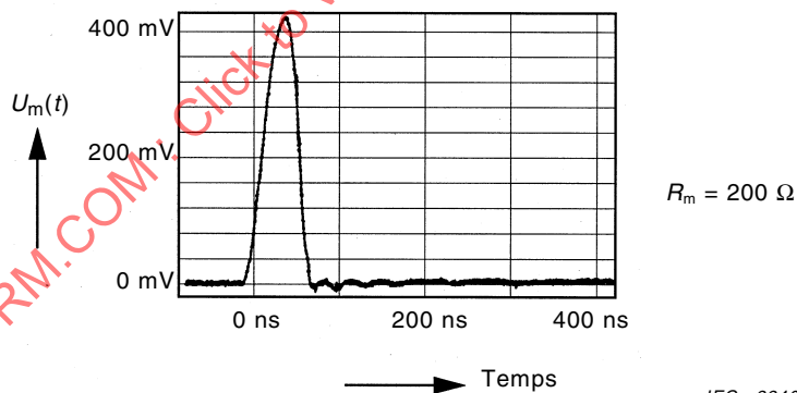
Figure A.1b – Impulsions d'étalonnage u_m(t) d'un calibre typique relié aux résistances de mesure R_m = 33 \Omega et R_m = 200 \Omega respectivement ( q = 100 \text{ pC} )
