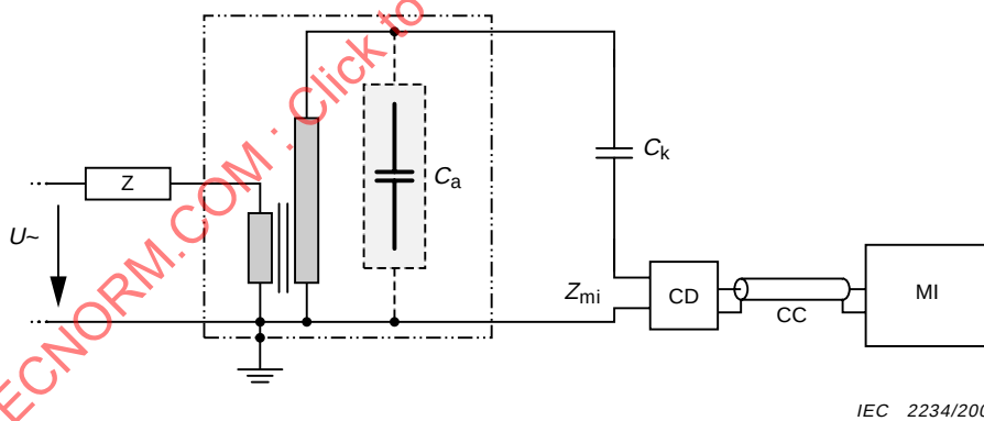
Figure 2 – Circuit d'essai pour une mesure faite à la prise d'une traversée
