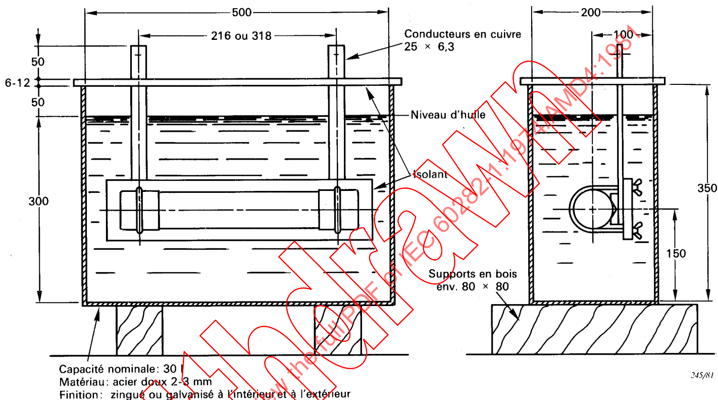
Cuve d'essai pour essais d'échauffement des fusibles immergés dans l'huile.
