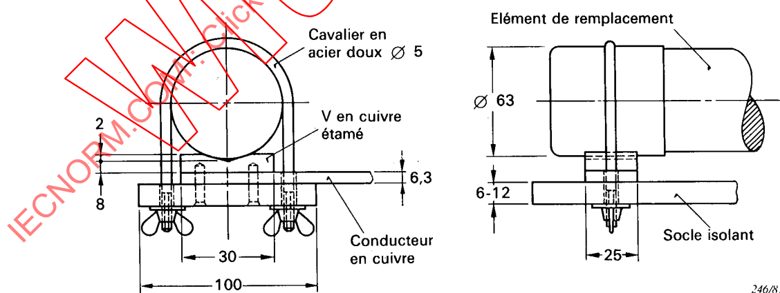
Détail de la fixation de l'élément de remplacement dans la cuve.
