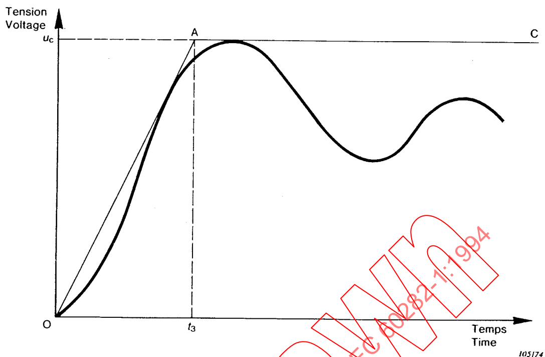
Figure 10 – Exemple d'un tracé de référence à deux paramètres pour une T.T.R. dont la partie initiale présente une concavité vers la gauche Example of a two-parameter reference line for a T.R.V. whose initial portion is concave towards the left
