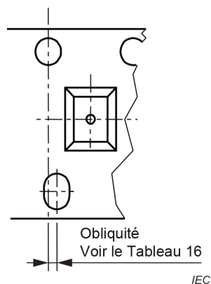
Figure 15 – Obliquité du trou d'entraînement allongé
