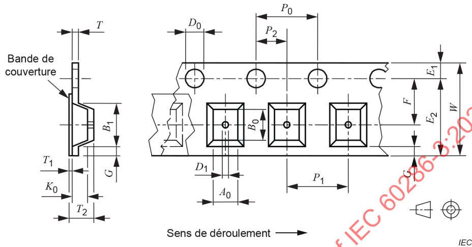
Figure 8 – Dimensions d'une bande d'entraînement gaufrée (8 mm, 12 mm, 16 mm et 24 mm)
