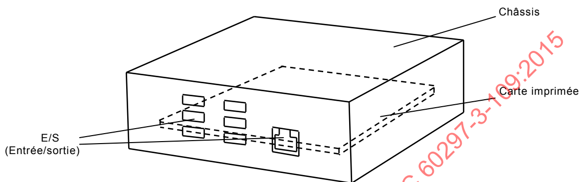
Figure 2 – Disposition d'un châssis dans une application intégrée
