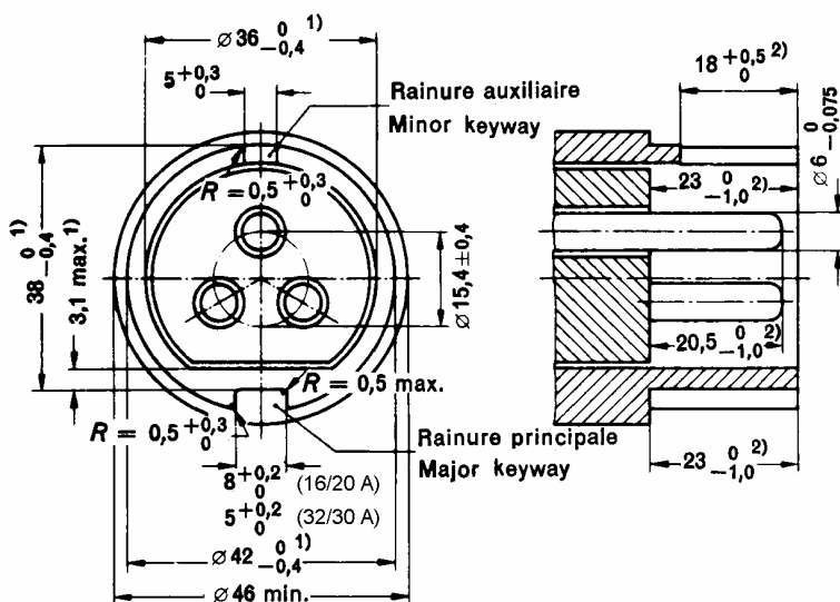
DISPOSITION DES BROCHES
