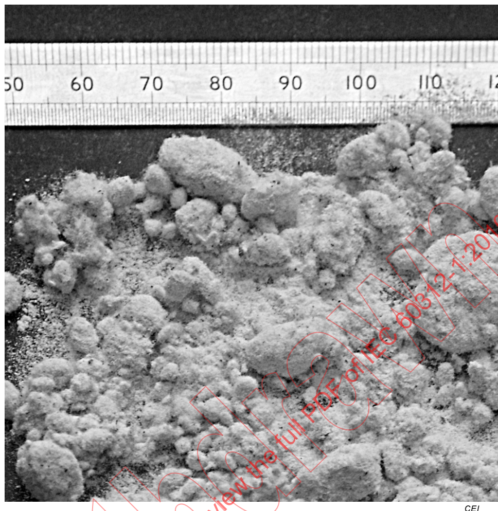
Figure 11 – Poussière d'essai pour le chargement du réservoir à poussière
