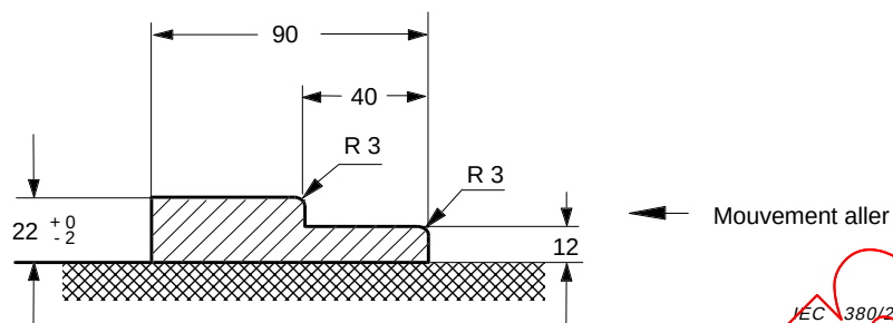
Figure 20A – Coupe du seuil
