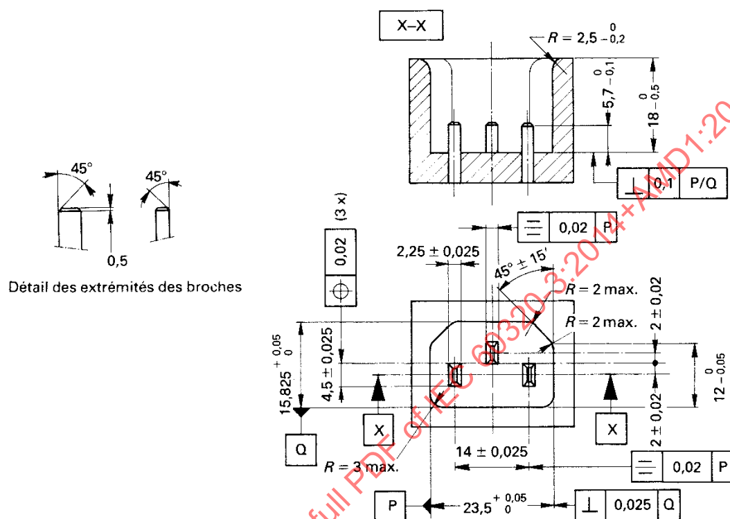
Figure 14 – Calibre "ENTRE" pour prises mobiles selon conformément à la feuille de norme C13
