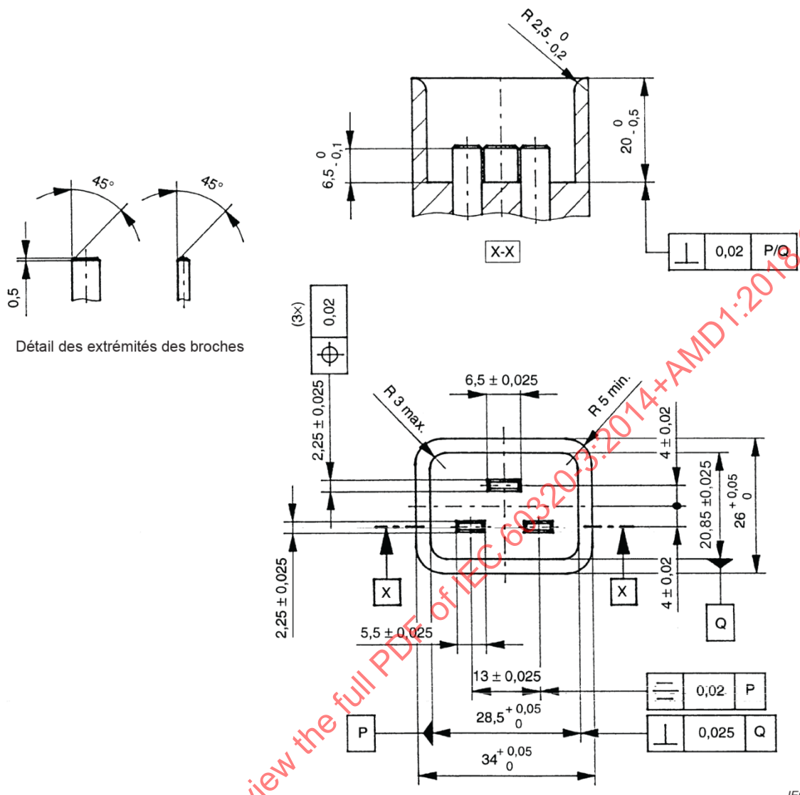
Figure 29 – Calibre "ENTRE" pour socles femelles de connecteurs selon conformément à la feuille de norme J
