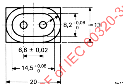
Figure 2 – Calibre "ENTRE" pour prises mobiles conformément à la feuille de norme C1
