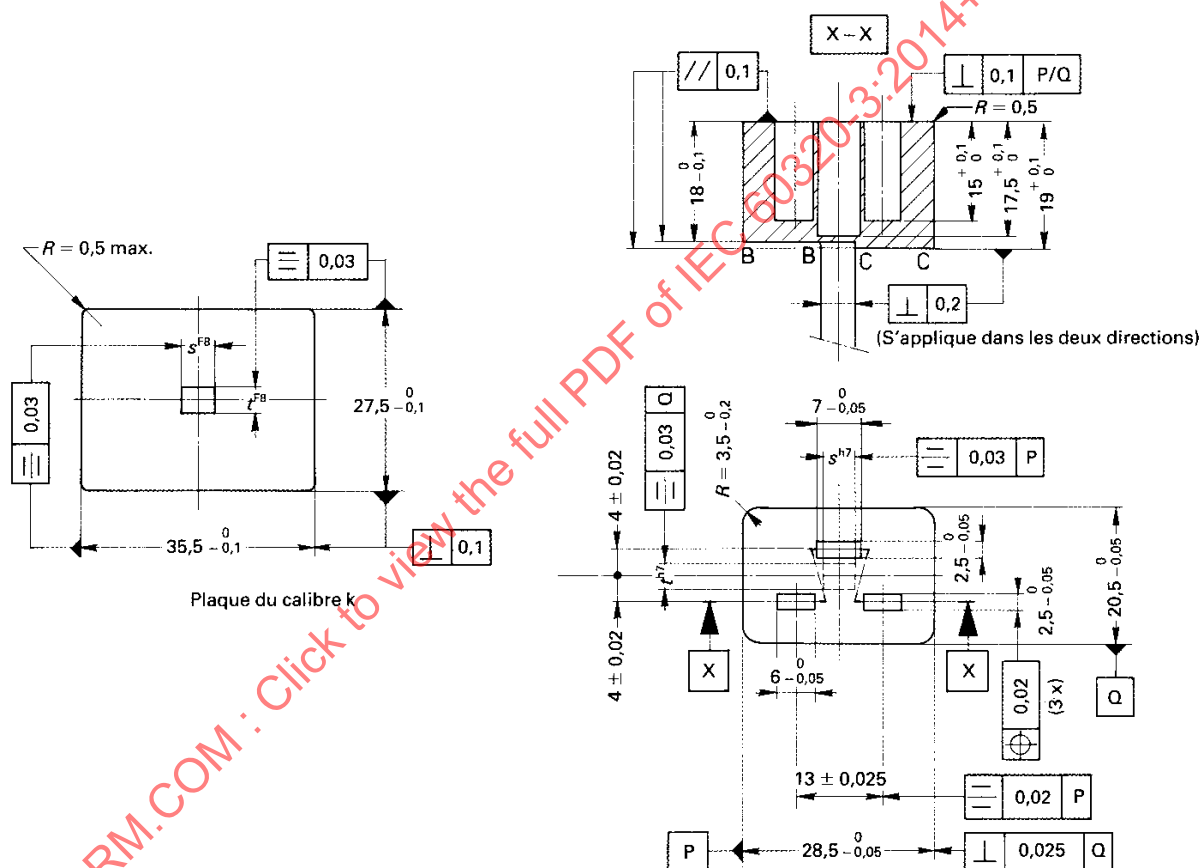
Figure 20 – Calibre "ENTRE" pour socles de connecteurs selon les conformément aux feuilles de norme C20 et C24
