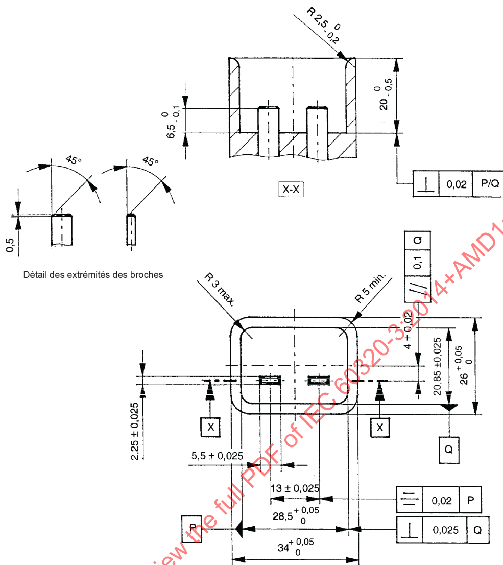
Figure 30 – Calibre "ENTRE" pour socles femelles de connecteurs selon conformément à la feuille de norme L
