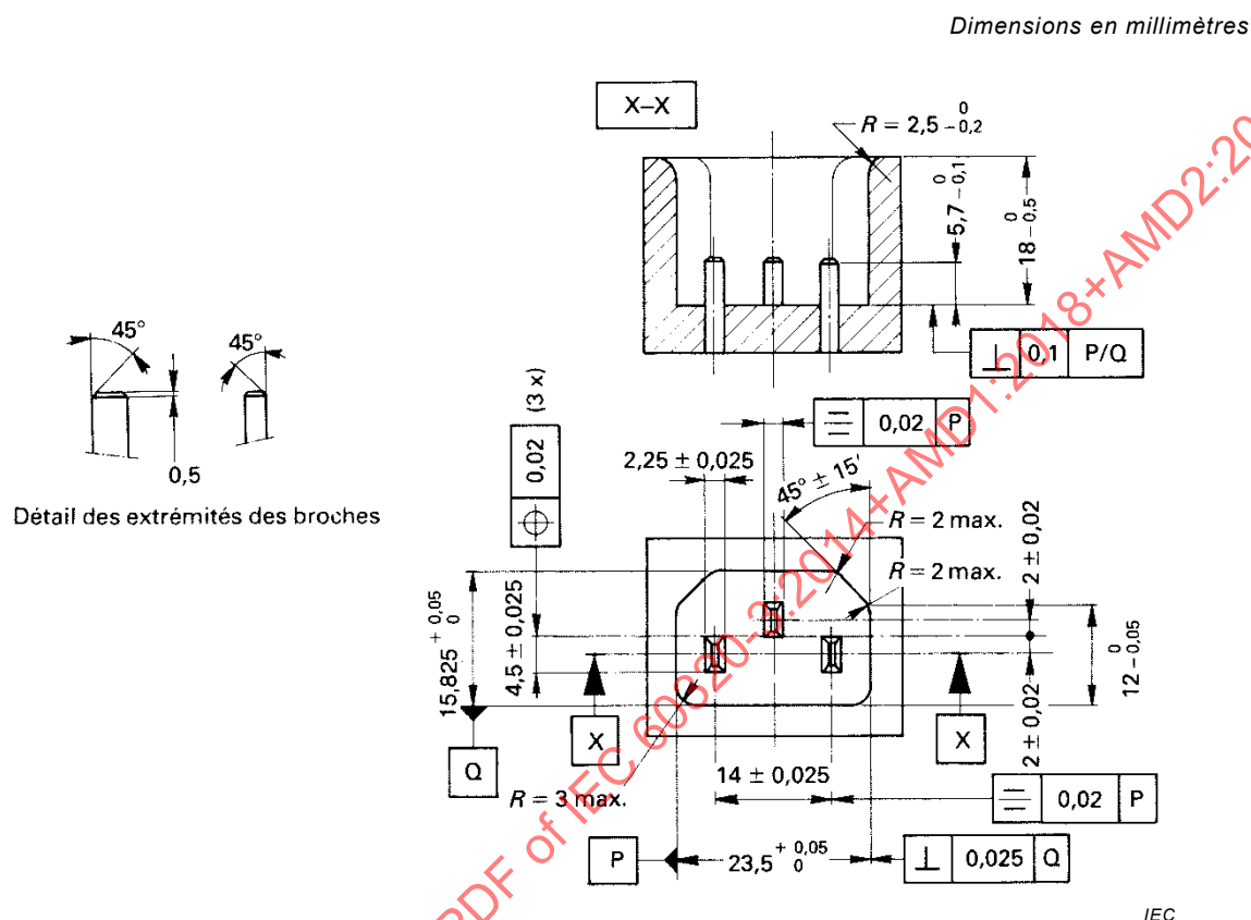
Figure 14 – Calibre "ENTRE" pour prises mobiles selon conformément à la feuille de norme C13
