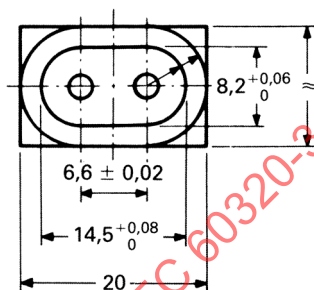
Figure 2 – Calibre "ENTRE" pour prises mobiles conformément à la feuille de norme C1
