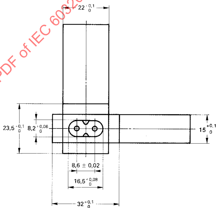
Figure 5 – Calibre "ENTRE" pour prises mobiles à entrées latérales selon conformément à la feuille de norme C7
