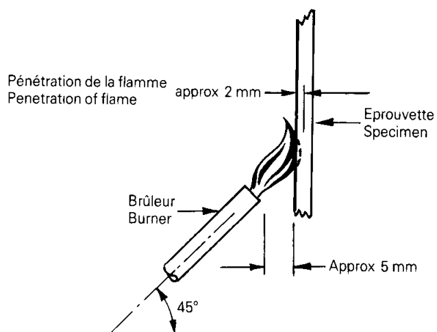
FIG. 1d. — Epreuve verticale. Côté bas horizontal. Flamme appliquée sur la surface. Specimen vertical. Lower edge horizontal. Flame applied to surface.
