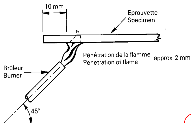
FIG. 1a. – Epreuve horizontale. Flamme appliquée sur la surface. Specimen horizontal. Flame applied to surface.
