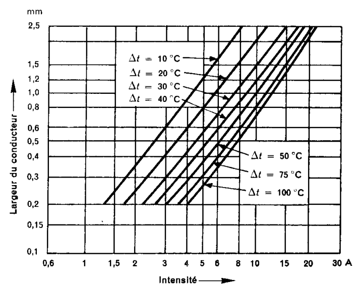
Épaisseur du conducteur 105 μm
