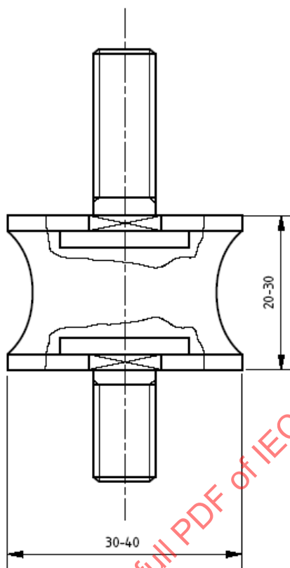
Figure 4 – Manchon amortisseur type en caoutchouc (dureté shore A 50-60) pour fixer le panneau d'essai
