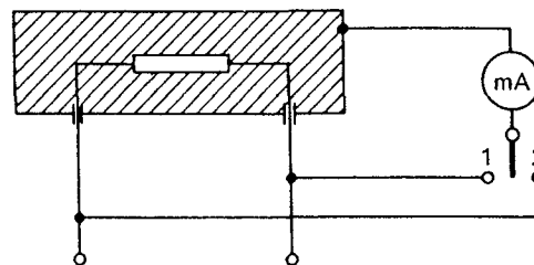
FIG. 5. — Schéma pour la mesure du courant de fuite à la température de régime pour connexion monophasée des appareils autres que ceux de la classe II. Diagram for leakage current measurement at operating temperature for single-phase connection of appliances other than those of Class II.
