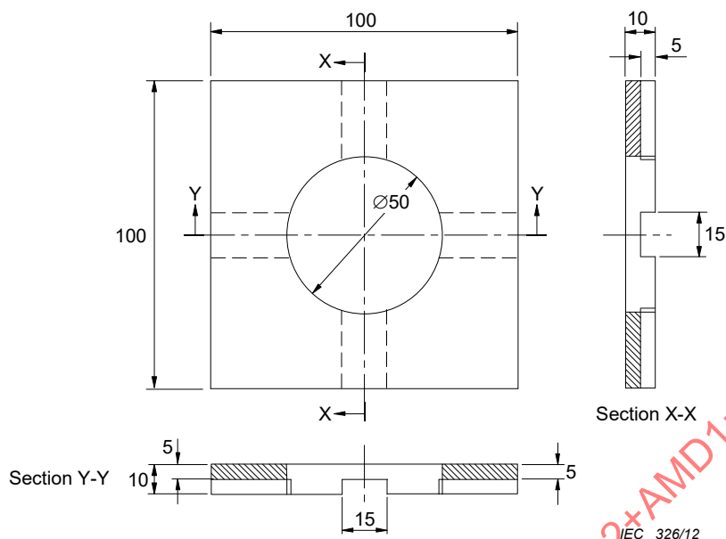
Figure 113a – Détail A – Partie inférieure du masque
