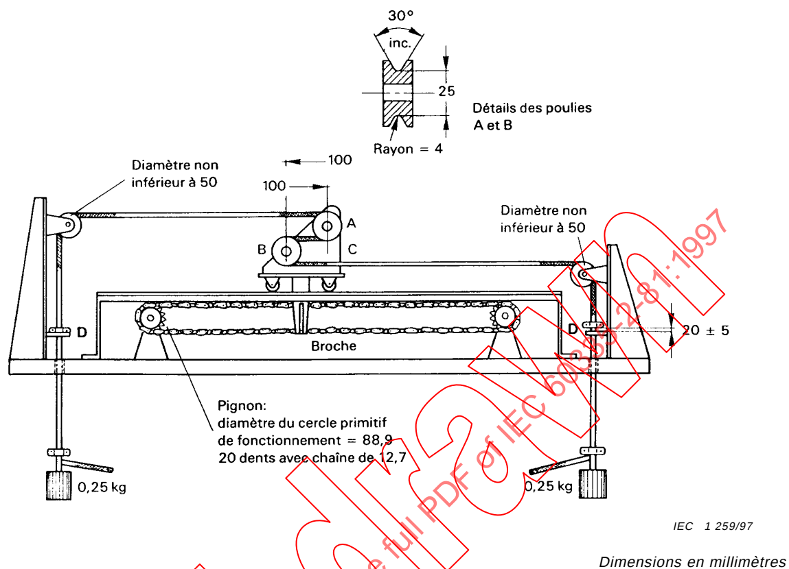
Figure 102 – Appareil pour l'essai de flexion des éléments chauffants et conducteurs internes
