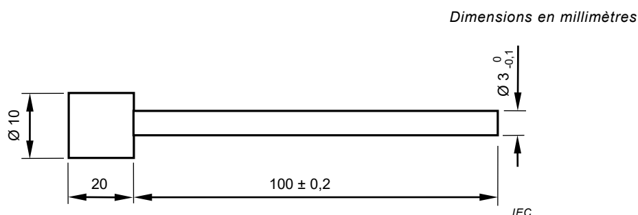
Figure 101 – Tige d'essai pour la dissimulation du verrouillage
