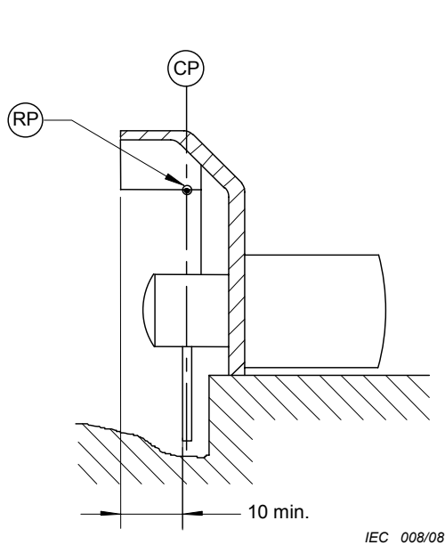
Figure 102a – Section partielle en AA (protecteur uniquement)
