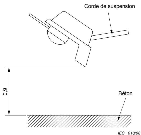
Figure 103 – Essai de résistance du protecteur (appareils portatifs)
