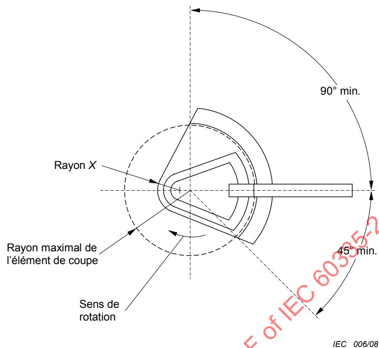
Figure 101a – Vue de dessus
