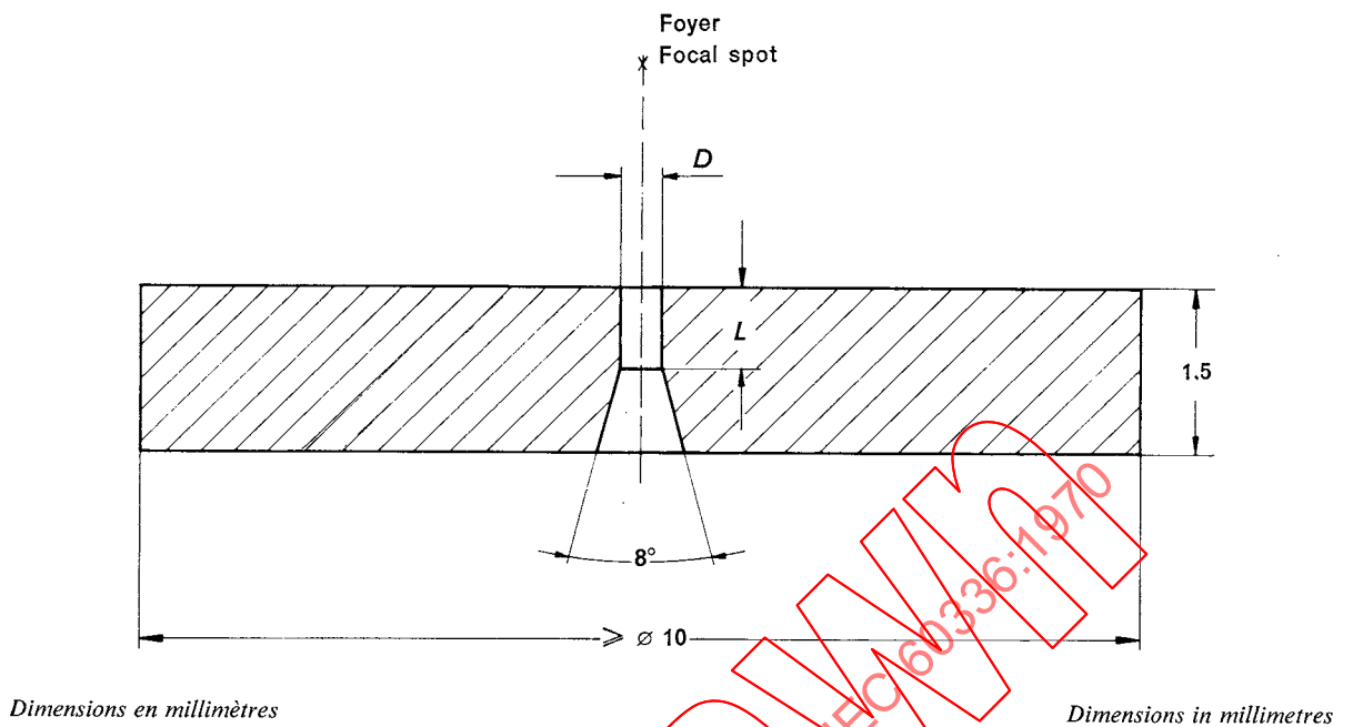
FIG. 1. — Coupe transversale du sténopé avec indication des dimensions essentielles. Cross-sectional view of the pinhole diaphragm indicating the essential dimensions.
