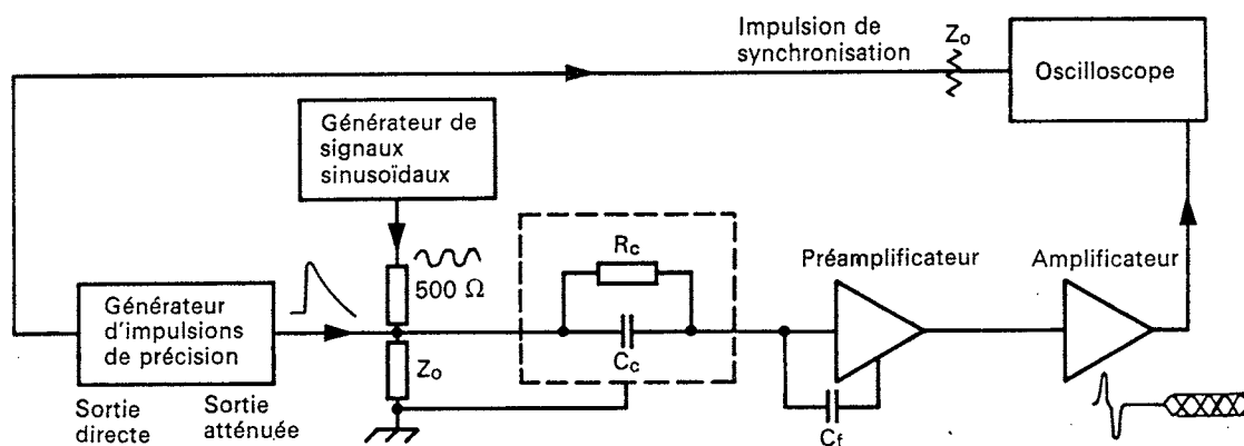
FIG. 18. — Mesure du temps de restitution du gain de l'amplificateur. (Mise en forme par double ligne à retard.)
