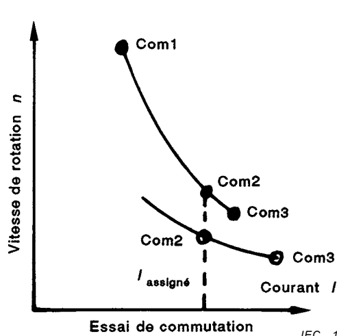
Figure 1c – Moteur de véhicule thermoélectrique
