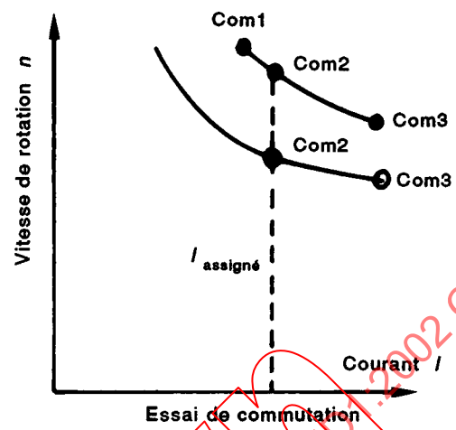
Figure 1a – Moteur série alimenté directement par une ligne de contact
