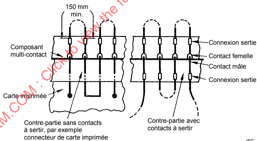
Figure 7c – Exemple de connexions serties avec contacts pour composant multi-contacts (par exemple bornier ou connecteur)
