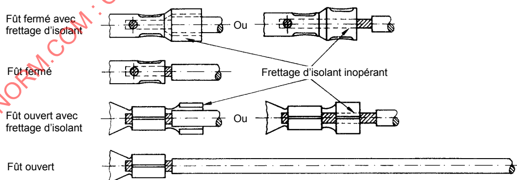
Figure 9 – Exemples de spécimens de type A
