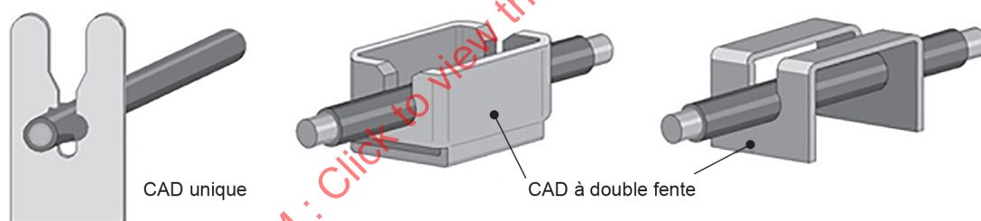
Figure 2 – Connexion autodénudante
