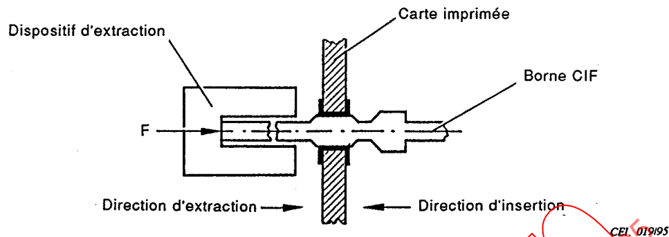
Figure 4 – Montage d'essai pour l'essai d'extraction
