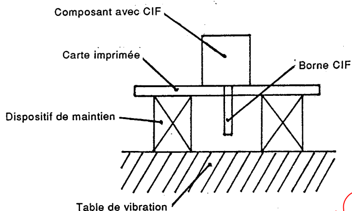
Figure 5 – Montage d'essai pour les vibrations
