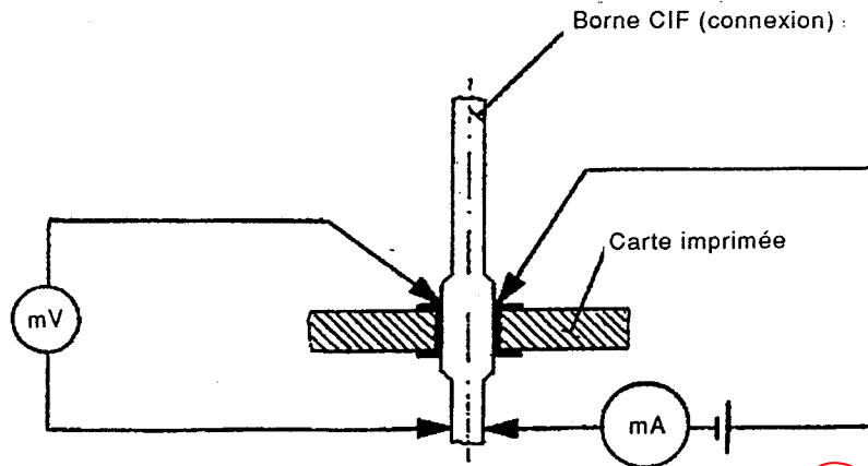
Figure 6 – Montage d'essai pour la résistance de contact
