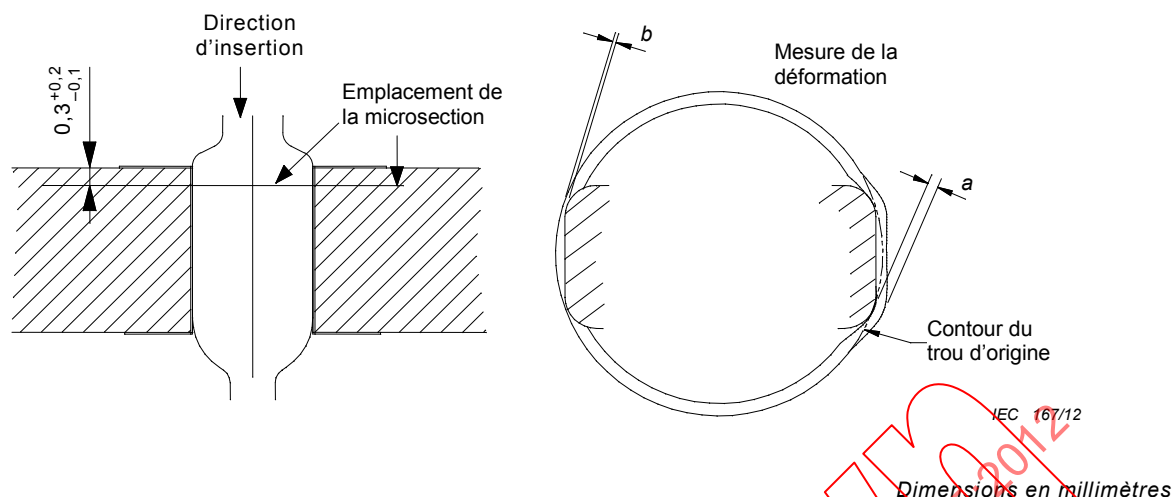
Figure 6 – Coupe transversale d'une connexion insérée à force
