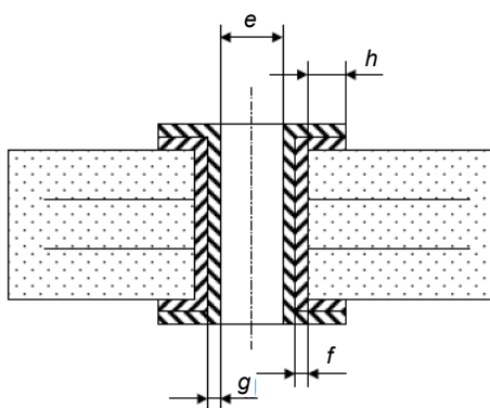
Figure 1 – Trou métallisé
