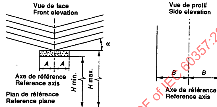
Eléments fixes du "box system" pour la vue de face et la vue de profil Fixed box system elements for front and side elevation
